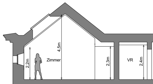
Schnitt B
