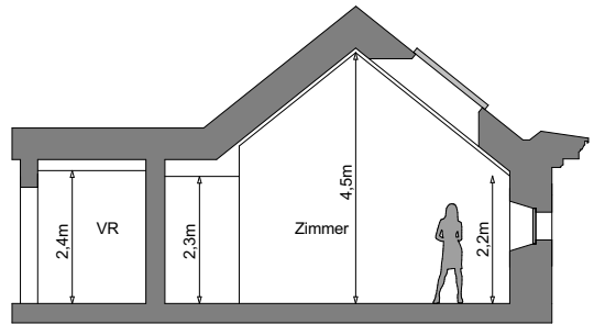
Schnitt B
